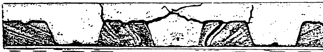
Fig. 5.4. Longitudinal rib shear failure.
